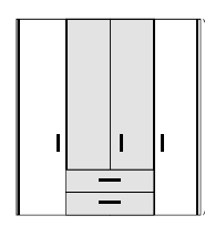
45 90 45 Breite = 180,1 cm
